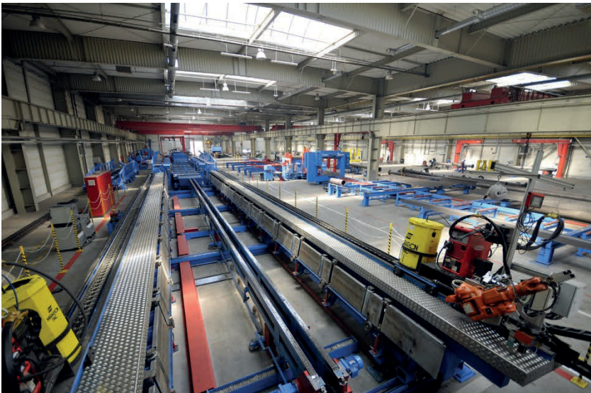
Produktionshalle mit Wellstegträger-Produktionslinie Production hangar with corrugated web beam production line
